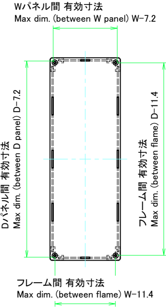
下カバー / Bottom cover
